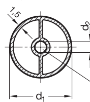
Ausführung für d_1 = 20 und 28
