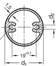
Ausführung für d_1 = 30
